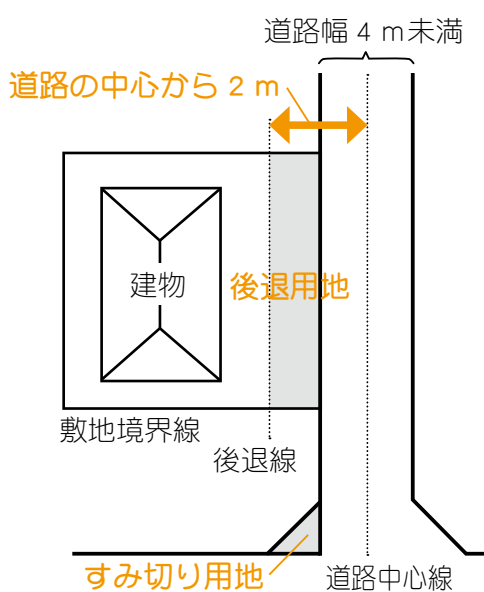
図1 後退用地とすみ切りの例
